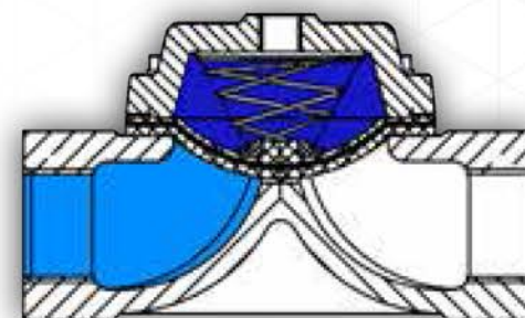
CON PRESIÓN EN LA CÁMARA, LA VÁLVULA CIERRA
